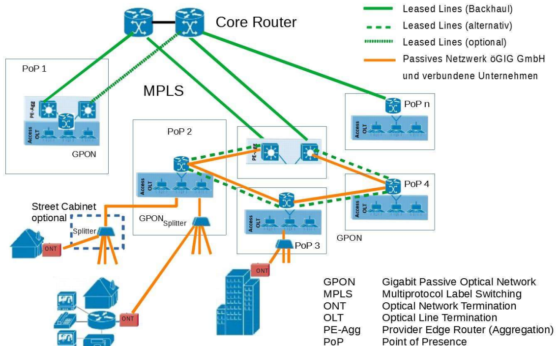
Abbildung 3 beispielhafte Netzwerktopologie
