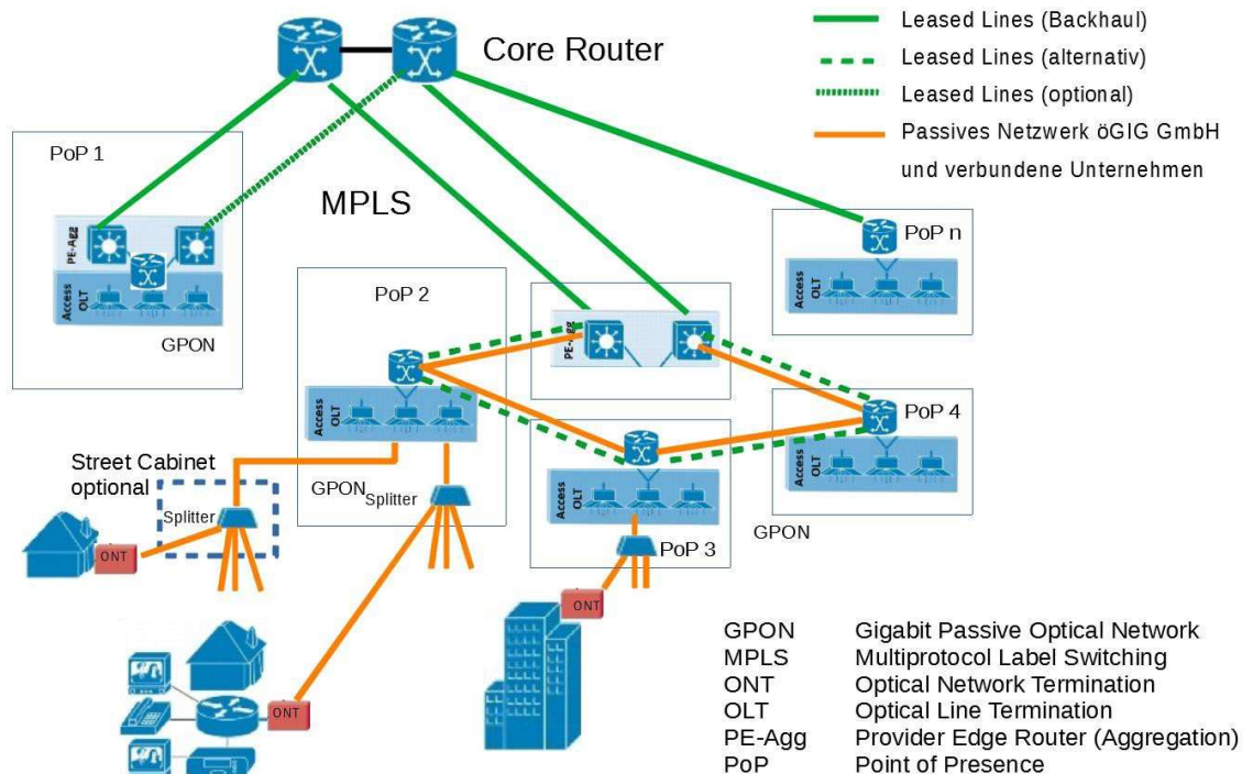
Abbildung 3 beispielhafte Netzwerktopologie
